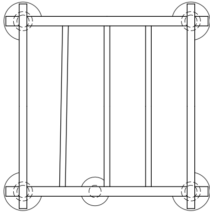
ESTRUCTURA DE SUELO
