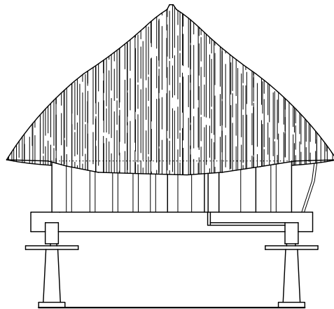
ALZADO NORTE
